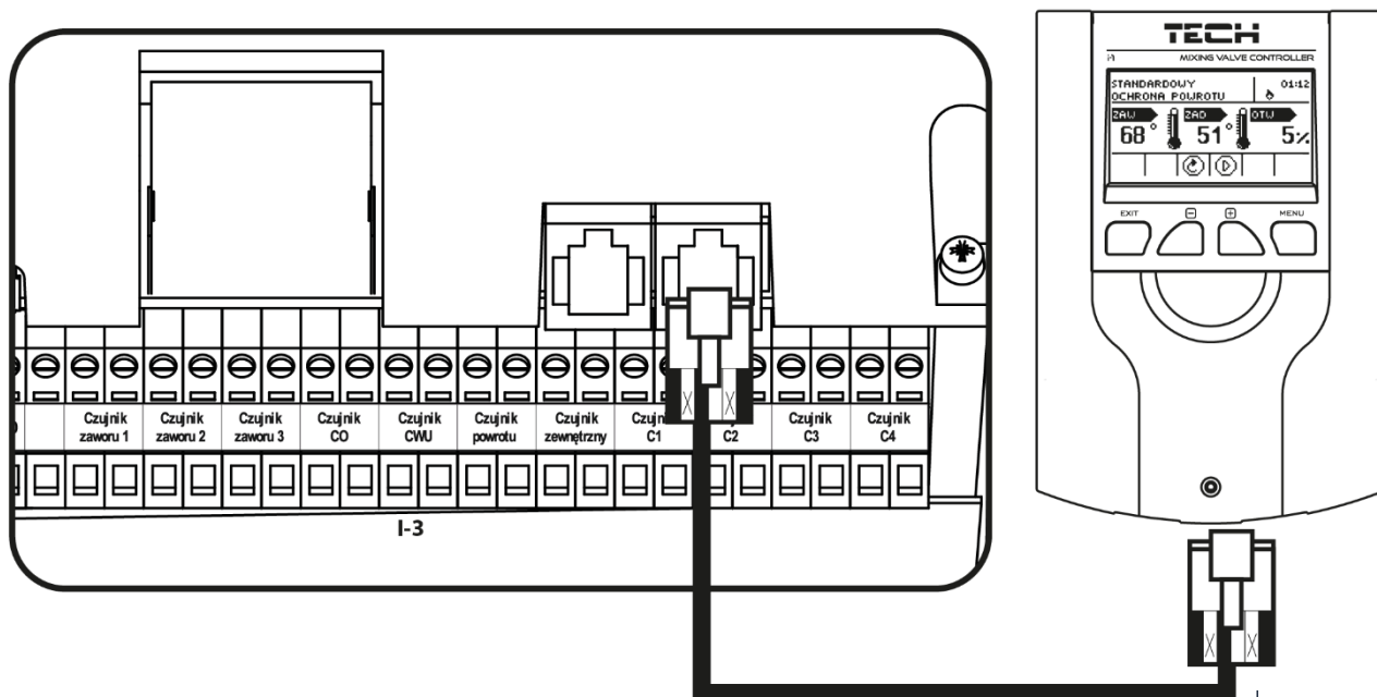
Przykładowe podłączenie zaworu dodatkowego ze sterownikiem głównym i-3
