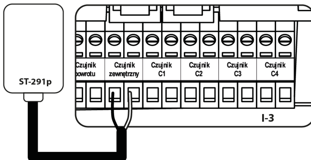
Podłączenie czujnika zewnętrznego
