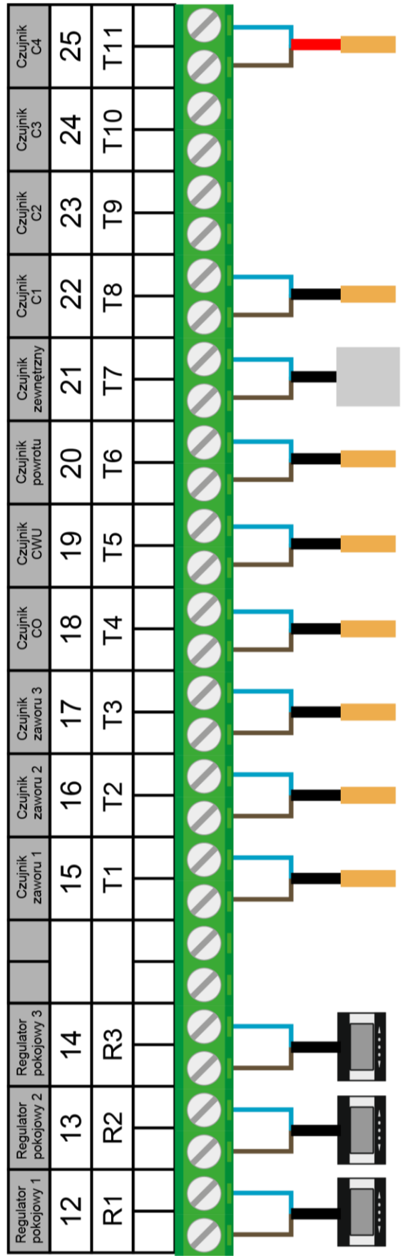
Złącza, symbole a przykładowe wykorzystanie
